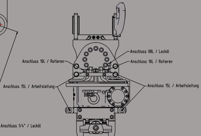
Ansicht ohne Schutzblech
