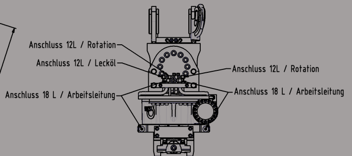
Ansicht ohne Schutzblech
