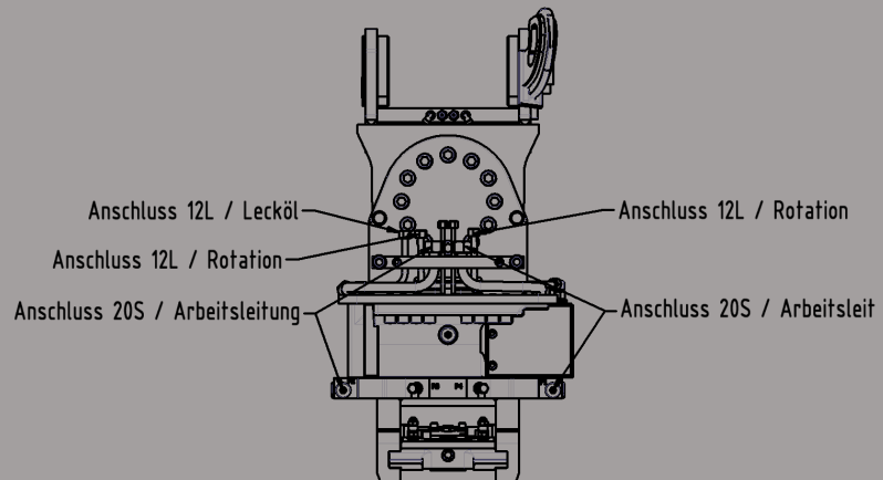
Ansicht ohne Schutzblech
